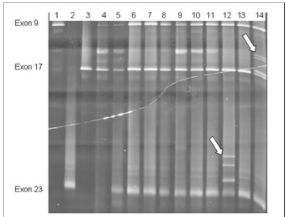
Obr. 1. Simultánní vyšetření exonů č. 9, 17 a 23 TSC1 genu metodou DGGE.
